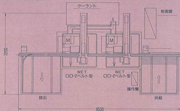
OD-2/2Hオートローダー装置付
