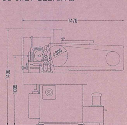
OD-2WET BELT標準機
